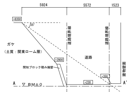
A~A' 断面图 S=1:200
